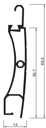
LP 55 EC2G
